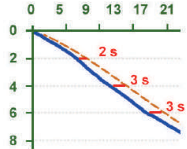
Figura 14: Taxa de afundamento dos anzóis em linhas secundárias do espinhel com pesos de 75 gramas posicionados a 5,5 metros dos anzóis e com o mesmo peso posicionado a 2 metros dos anzóis. Nota-se que com peso a 2 metros, os anzóis afundam mais rápido principalmente nos primeiros metros de profundidade que são os mais importantes para as aves marinhas.
