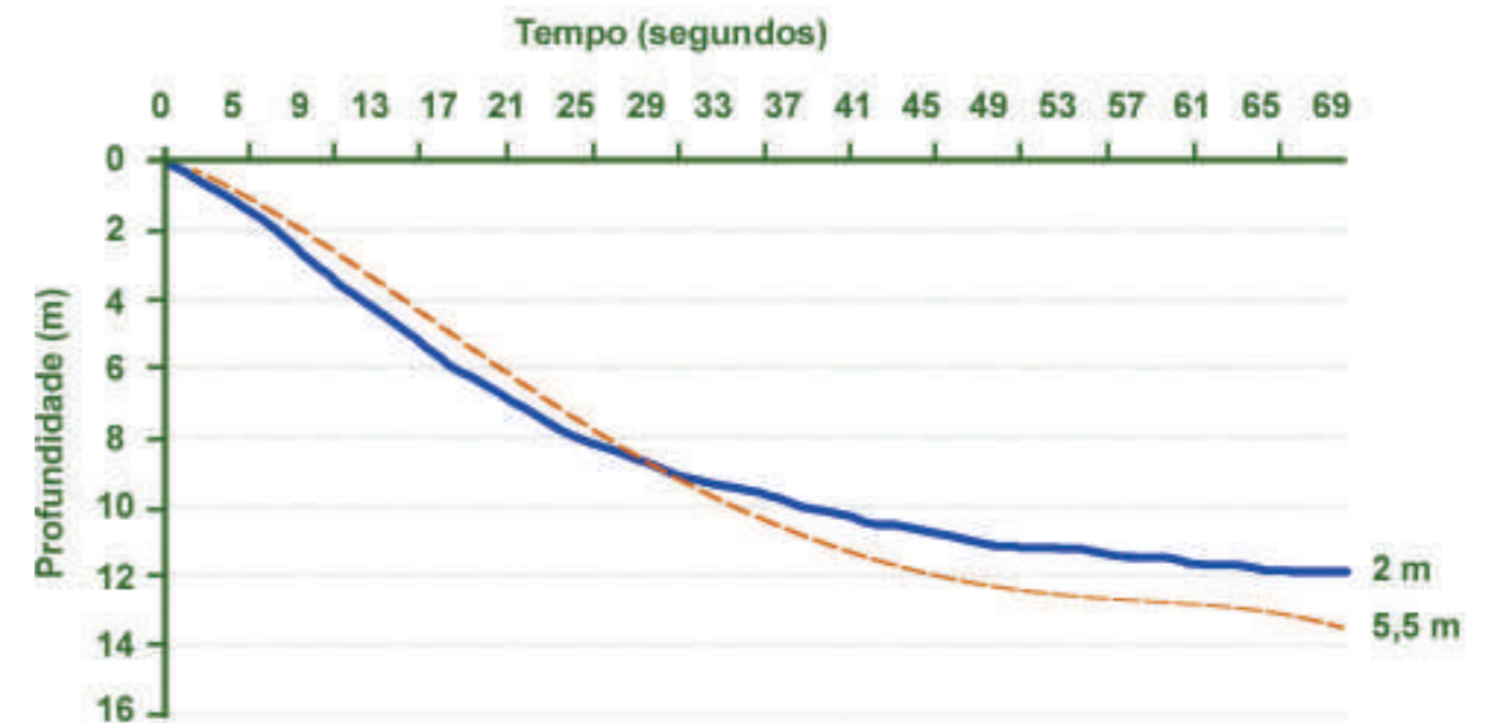
Figura 14: Taxa de afundamento dos anzóis em linhas secundárias do espinhel com pesos de 75 gramas posicionados a 5,5 metros dos anzóis e com o mesmo peso posicionado a 2 metros dos anzóis. Nota-se que com peso a 2 metros, os anzóis afundam mais rápido principalmente nos primeiros metros de profundidade que são os mais importantes para as aves marinhas.
