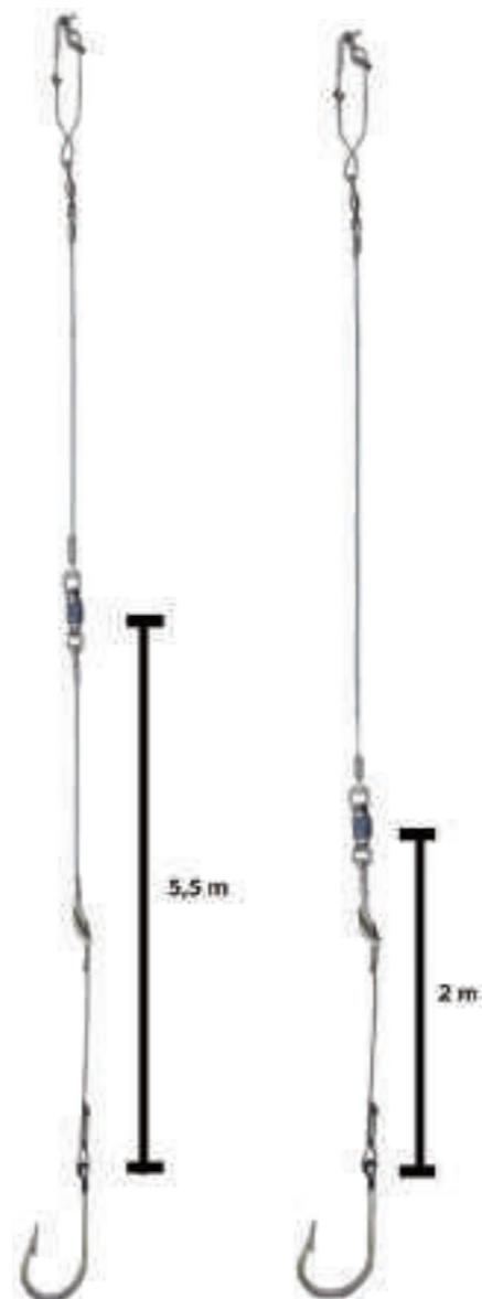
Figura 13: Configuração das linhas secundárias do espinhel pelágico com pesos de 60 gramas a 5,5 metros do anzol (configuração normalmente utilizada pelos pescadores) e com pesos de 60 gramas a 2 metros do anzol (para afundar mais rápido e reduzir a interação com as aves).
